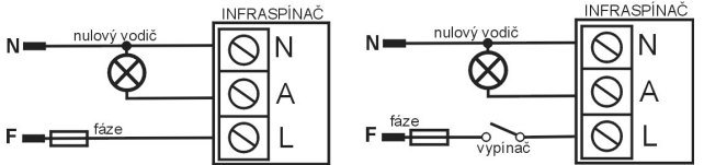
Zapojení bez vypínače
