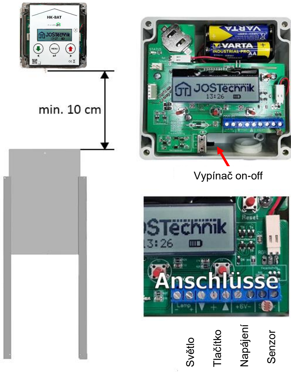
Obrázek: montáž samostatného zařízení
